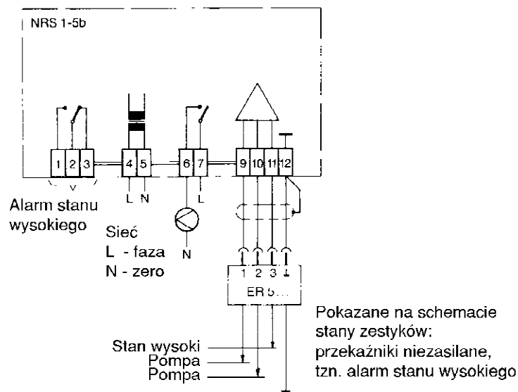
Rys. 3 Schemat połączeń regulatora poziomu NRS1-5b
